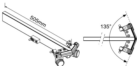
Scatola 087 AAP compl. 45°, L=505 RD Compl. 087 45° Open Corner case L=505 RD
